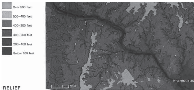
RELIEF
